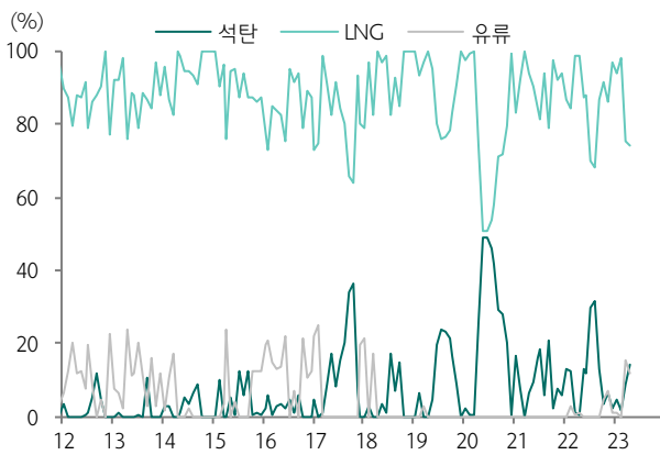
도표 3. 연료원별 SMP 결정비중 (4월 기저전원비중 14.3%)
